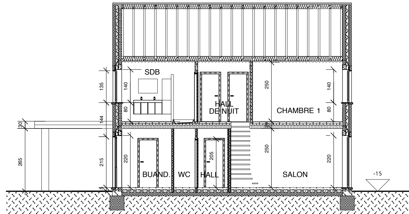
COUPE CC
