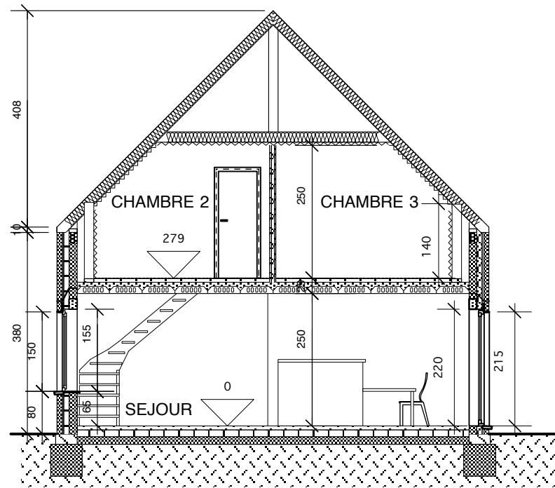
COUPE AA
