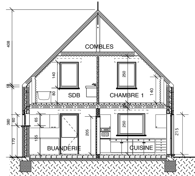
COUPE BB
