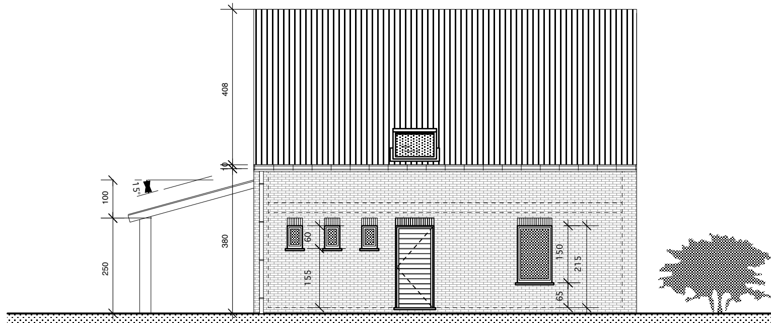
FACADE AVANT
